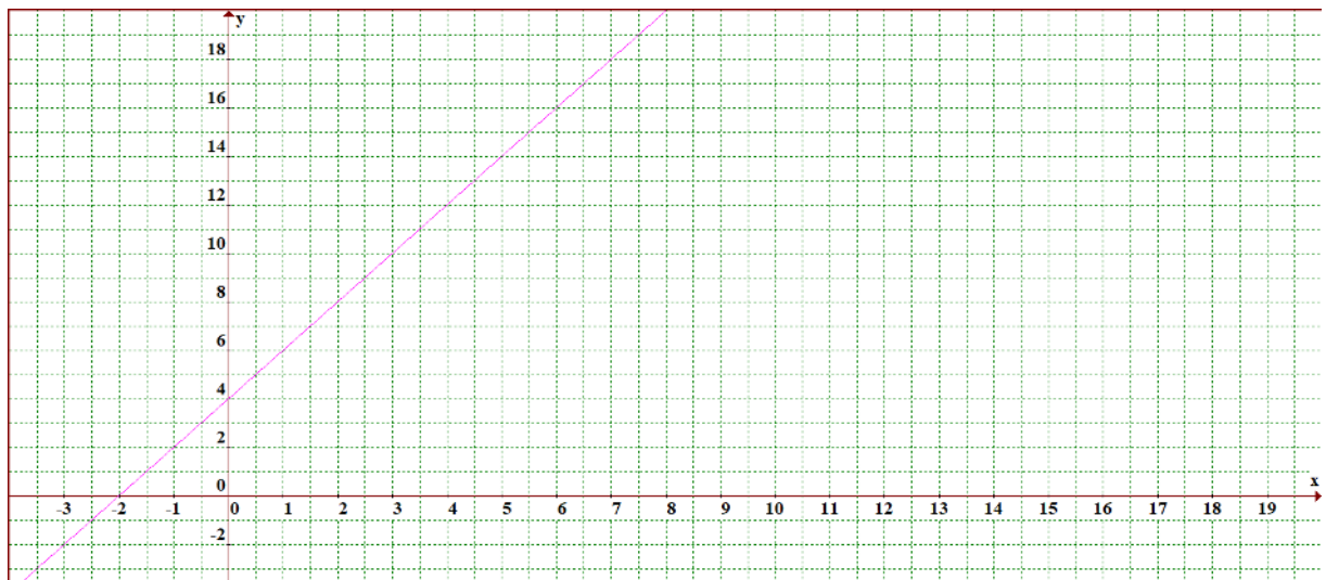
Gráfico 1 - Representação gráfica da função f(x)=2x+4
