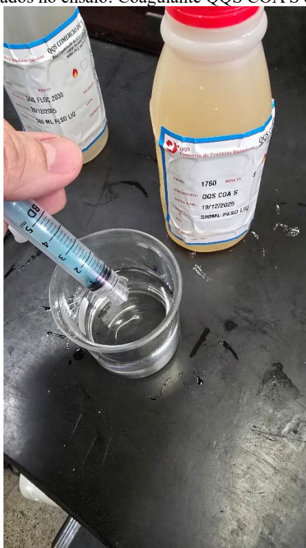
Figura 1: Produtos avaliados no ensaio: Coagulante QQS COA S e Floculante QQS FLOC.
