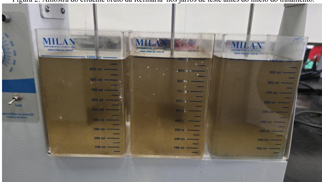
Figura 2: Amostra do efluente bruto da Refinaria nos jarros de teste antes do início do tratamento.
